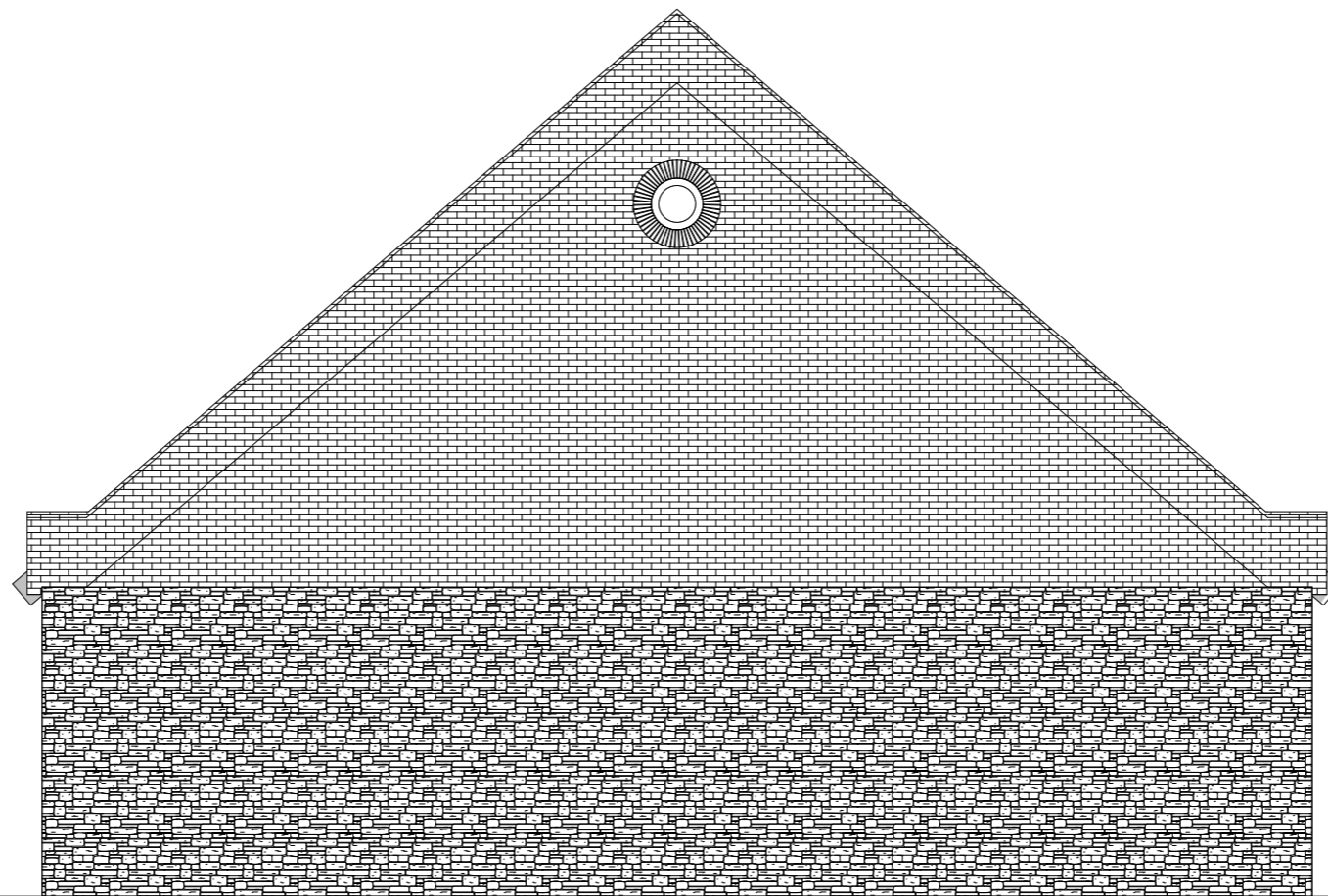
Ansicht Ost
