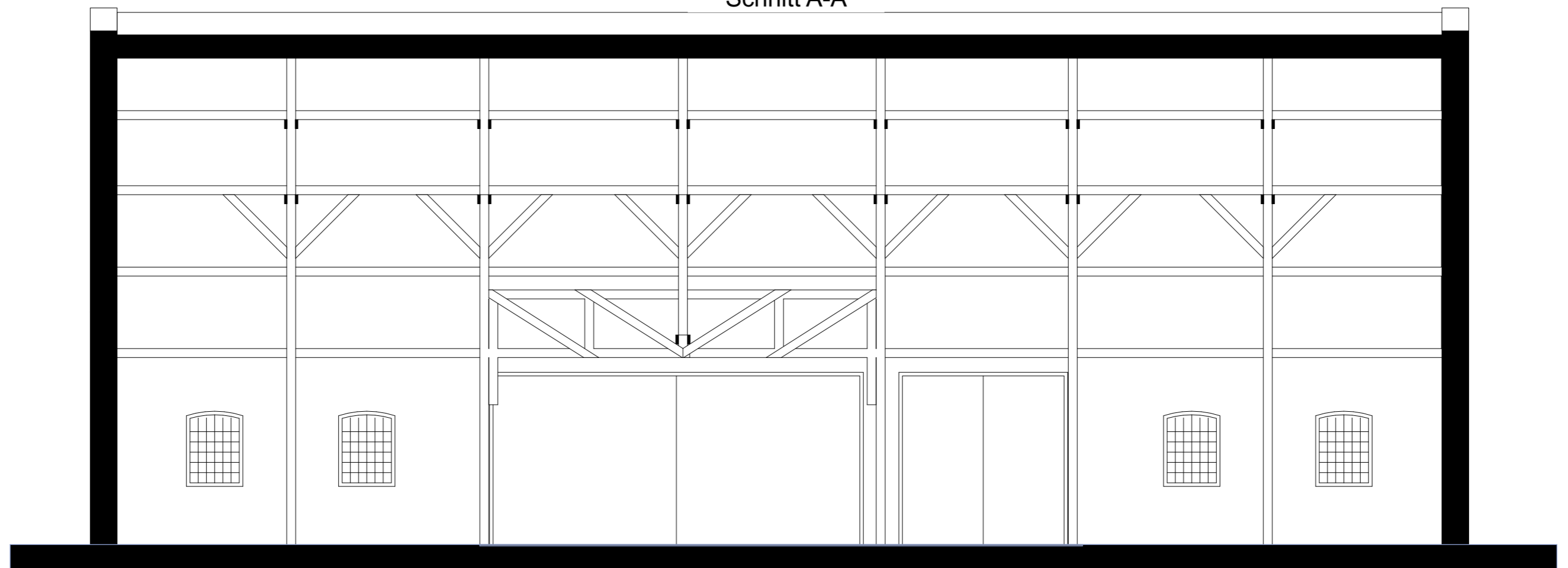
Schnitt B-B
