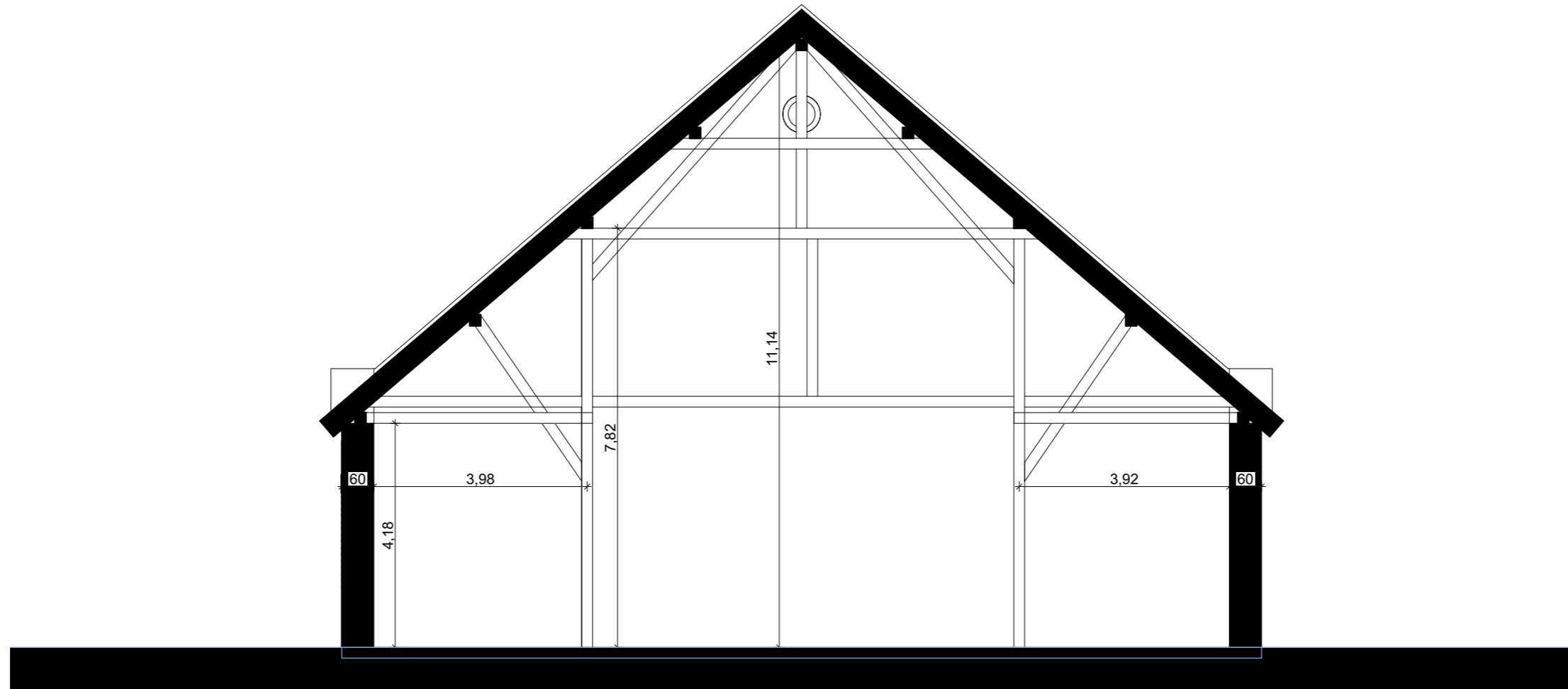
Schnitt A-A
